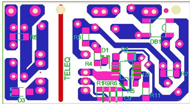
Bottom layer of PCB
