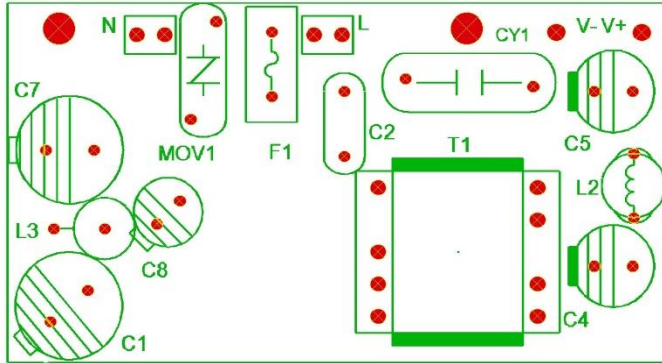
Top layer of PCB
